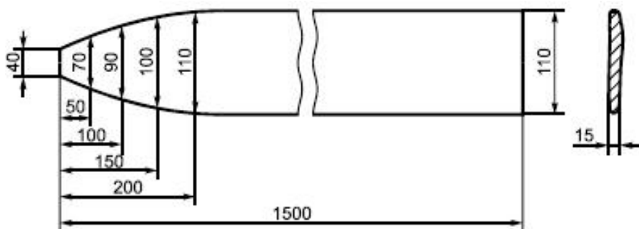
Рисунок 1 - Правилка А
